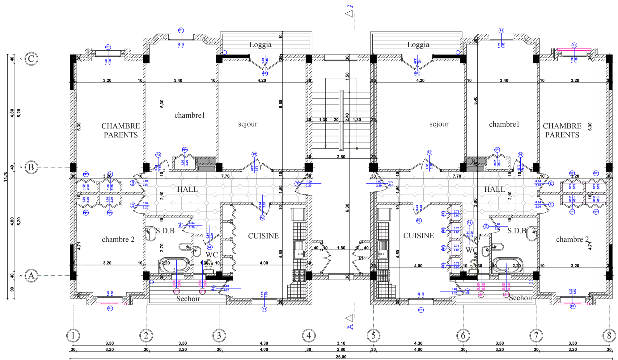
PLAN ETAGE COURANT
