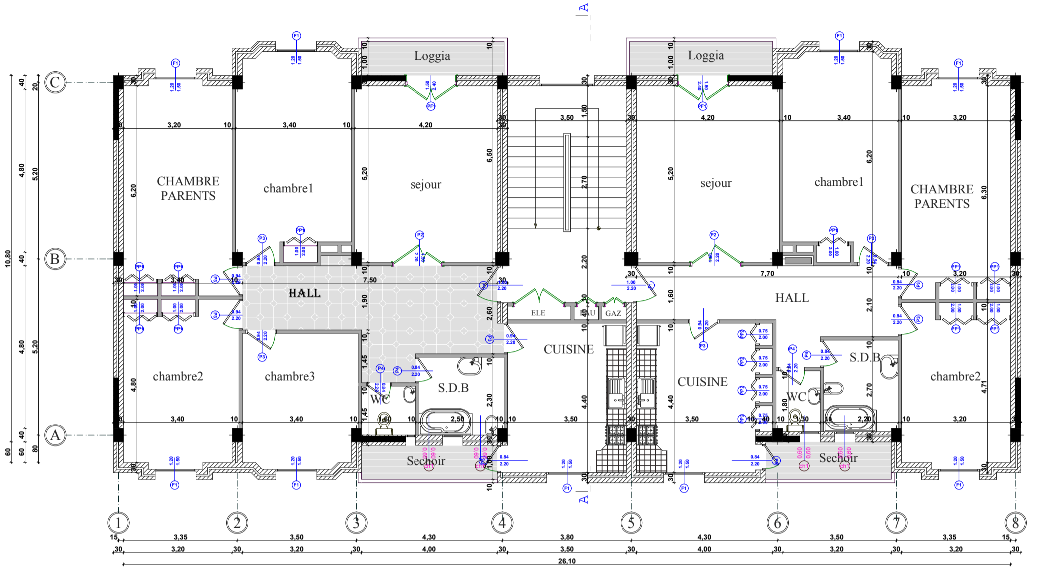
PLAN ETAGE COURANT
