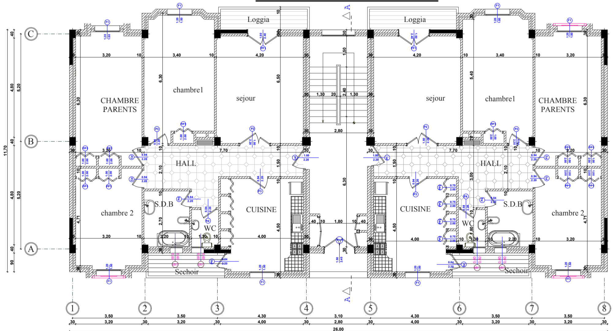
PLAN DU RDC
