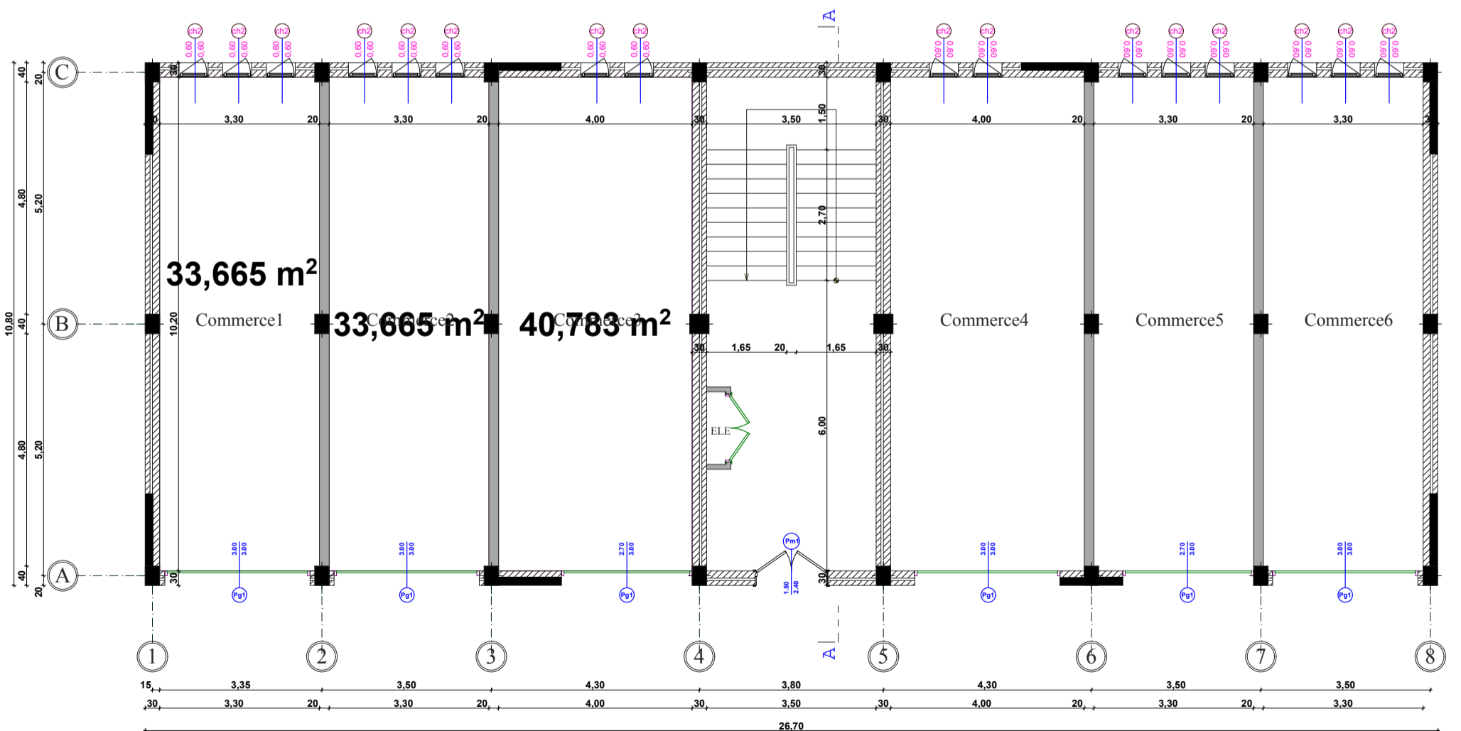
PLAN DU RDC
